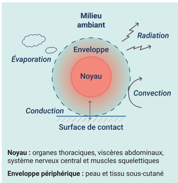
Figure 1 : Différentes modalités d'échange thermique entre le milieu ambiant et l'organisme
